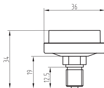
M10*1 (L型)
